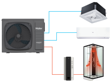
Provoz 5: Příprava teplé vody + chlazení
