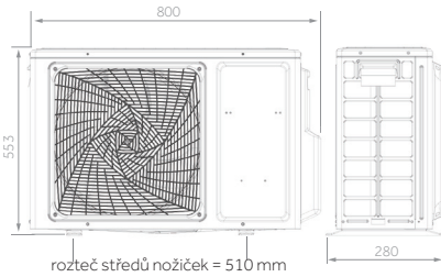
1U25 / 1U35
