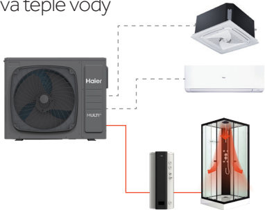
Provoz 1 Příprava teplé vody
